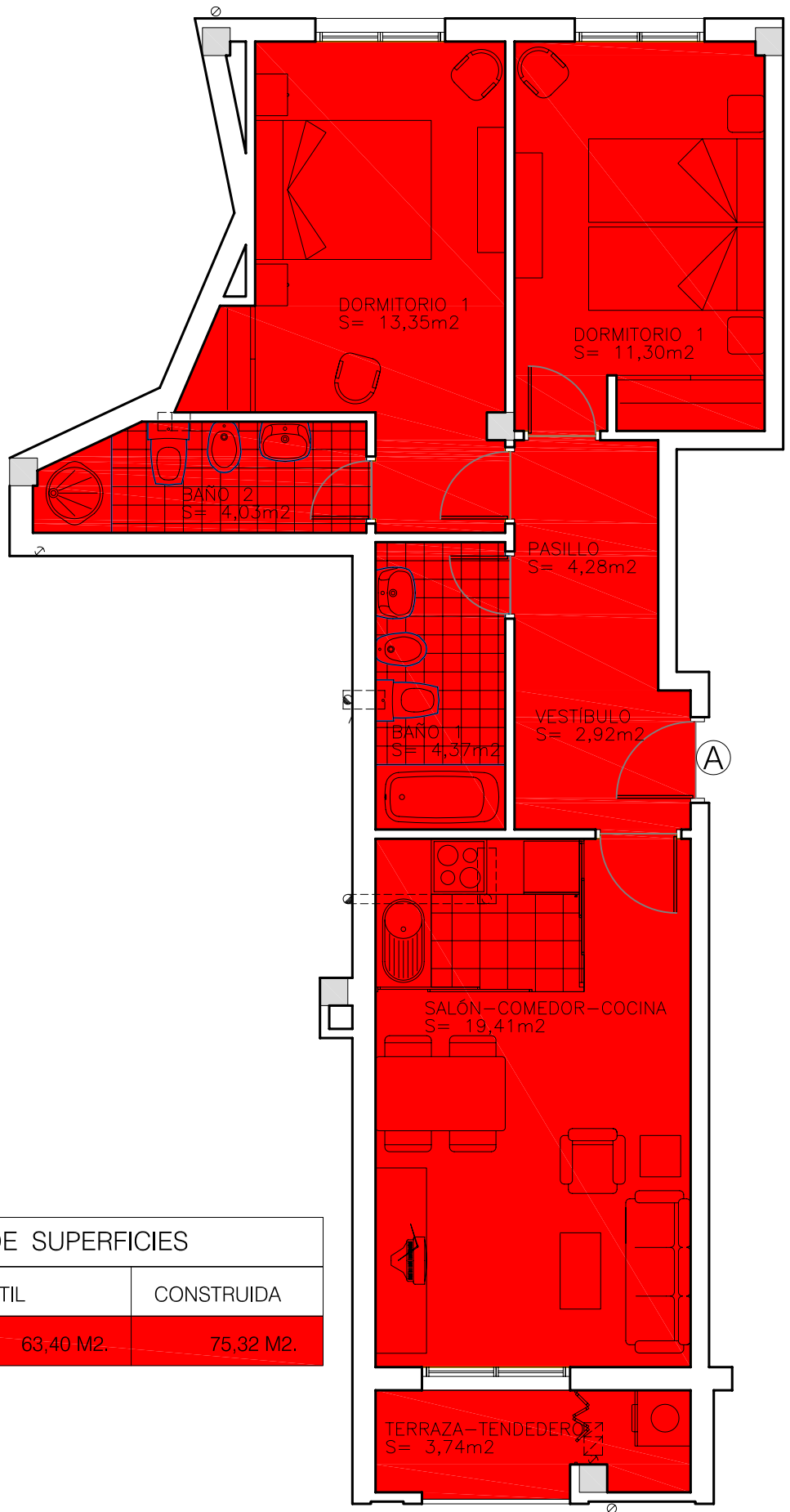
PLANTA BAJA. VIVIENDA TIPO "A"
