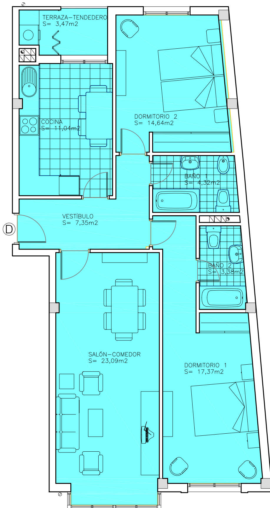
PLANTA SEGUNDA. VIVIENDA TIPO "D"
